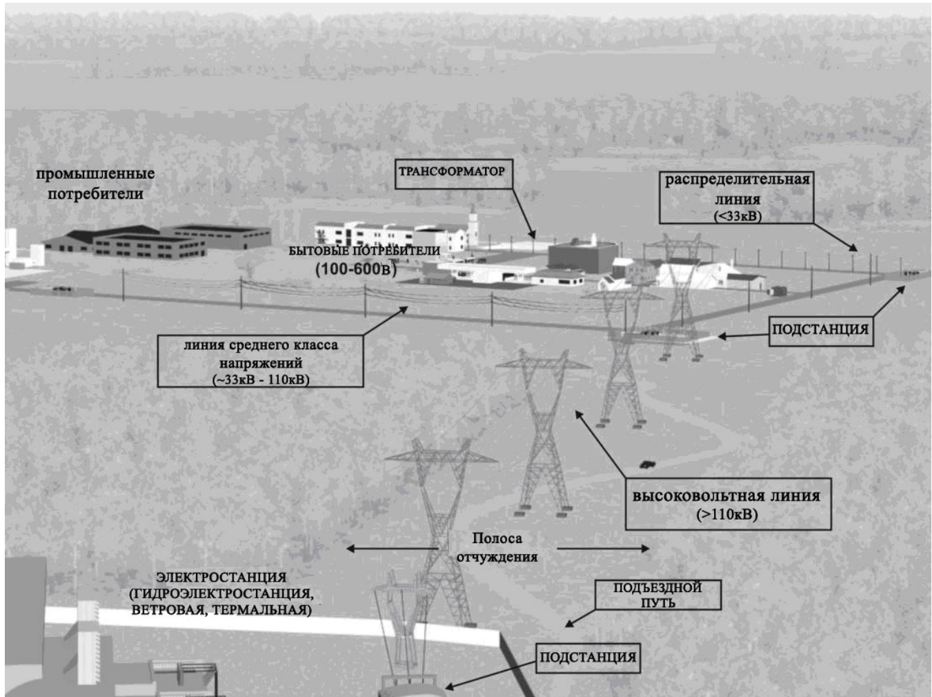
Рис. А-1: Передача и распределение электроэнергии
